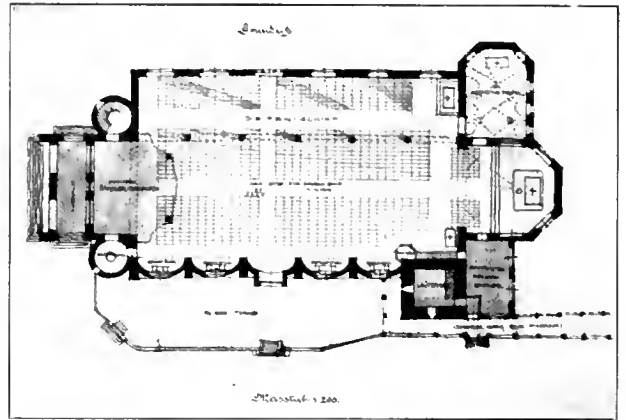
MOLTO ZWISCHENTIGG GRUNDRIß Nr. 12, Blatt S. VII - X, zgl. Nr. 13 - 15
